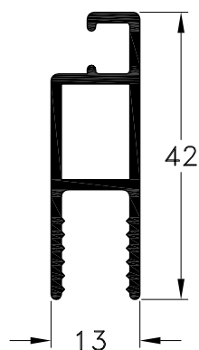
1020685 - Mosquitero Peso: 0,38 Kg/m. Largo Std.: 6.030 mm.
