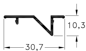
1040509 - Tapa Peso: 0,14 Kg/m. Largo Std.: 6.030 mm.
