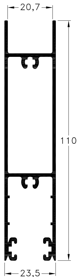
1020686 - Zócalo D.V.H. Puerta Corrediza Peso: 1,23 Kg/m. Largo Std.: 6.030 mm.
