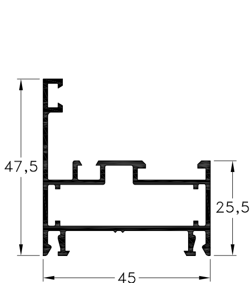
1020662 - Marco Peso: 0,71 Kg/m. Largo Std.: 6.150 mm.
