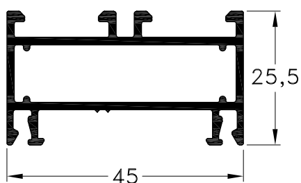
1020621 - Zócalo Bajo Peso: 0,67 Kg/m. Largo Std.: 6.030 mm.
