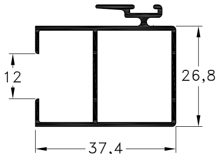
1020654 - Parante Central V.S. Peso: 0,58 Kg/m. Largo Std.: 6.150 mm.
