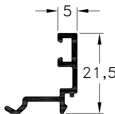
1020644 - Contravidrio Recto Exterior Puerta Peso: 0,18 Kg/m. Largo Std.: 6.030 mm.
