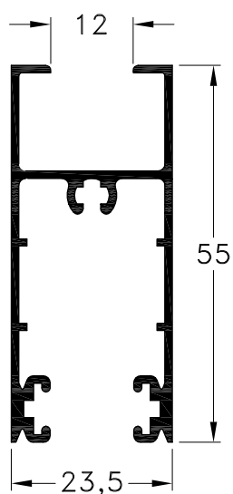
1020652 - Zócalo y Cabezal V.S. Peso: 0,64 Kg/m. Largo Std.: 6.030 mm.
