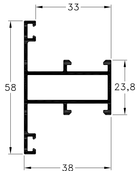
1020951 - Travesaño Angosto para Marco 1020656 Peso: 0,71 Kg/m. Largo Std.: 6.030 mm.
