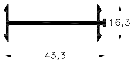
1020720 - Acople Recto Peso: 0,26 Kg/m. Largo Std.: 6.150 mm.
