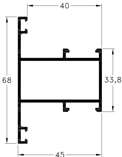
1020949 - Travesaño Ancho para Marco 668 Peso: 0,87 Kg/m. Largo Std.: 6.030 mm.
