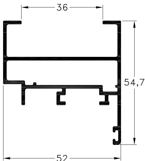
1020936 - Hoja Postigón Celosía Fija Peso: 0,88 Kg/m. Largo Std.: 6.150 mm.
