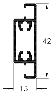
1020620 - Travesaño Mosquitero Peso: 0,45 Kg/m. Largo Std.: 6.030 mm.
