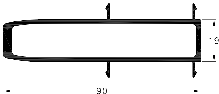
1020634 - Acople Columna Reforzado Peso: 1,24 Kg/m. Largo Std.: 6.150 mm.
