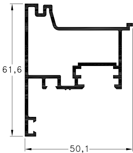
1020636 - Encuentro Central Peso: 0,92 Kg/m. Largo Std.: 6.150 mm.
