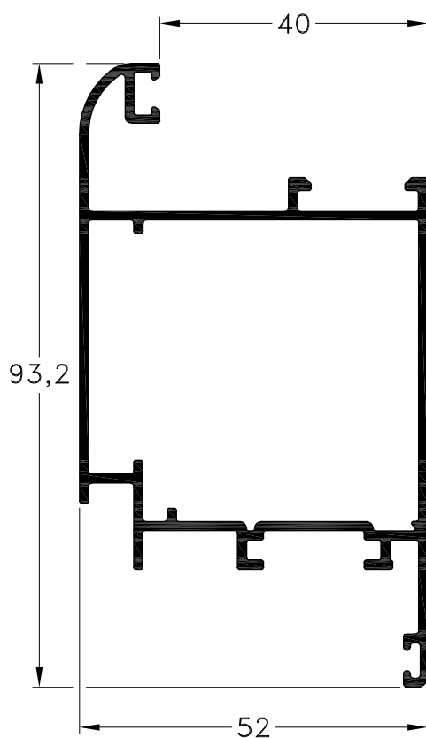
1020614 - Parante Peso: 1,15 Kg/m. Largo Std.: 6.150 mm.
