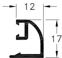
1020672 - Contravidrio Curvo Exterior Puerta Peso: 0,18 Kg/m. Largo Std.: 6.030 mm.
