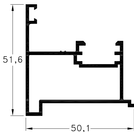
1020694 - Encuentro Central Ventana y Puerta de Abrir D.C. Peso: 0,80 Kg/m. Largo Std.: 6.150 mm.
