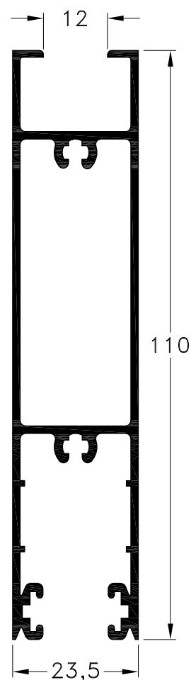
1020660 - Zócalo V.S. Puerta Corrediza Peso: 1,26 Kg/m. Largo Std.: 6.030 mm.
