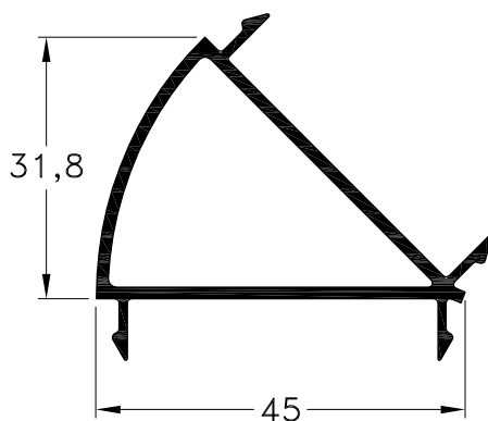
1020659 - Columna Curva a 45° Peso: 0,54 Kg/m. Largo Std.: 6.150 mm.
