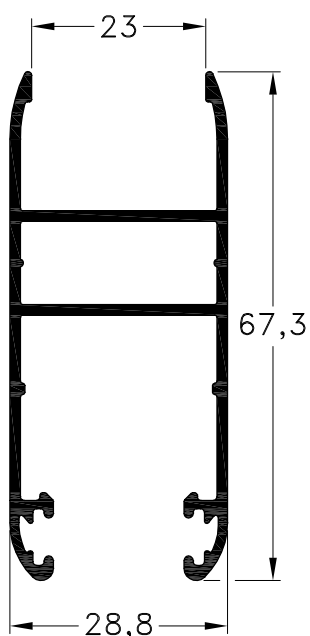
1020362 - Hoja Perimetral D.V.H. Peso: 0,80 Kg/m. Largo Std.: 6.150 mm.
