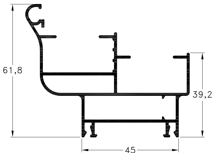
1020643 - Marco Peso: 1,10 Kg/m. Largo Std.: 6.030 mm.
