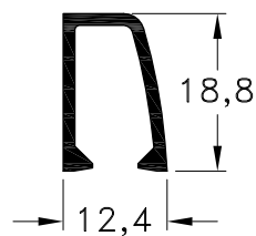
1020708 - Tope Mosquitero Peso: 0,19 Kg/m. Largo Std.: 6.030 mm.
