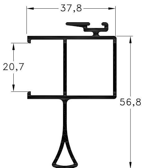
1020687 - Parante Central D.V.H. con Tirador Peso: 0,76 Kg/m. Largo Std.: 6.150 mm.
