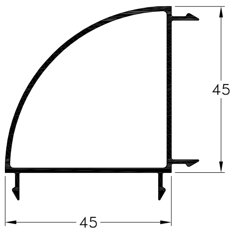
1020658 - Columna Curva a 90° Peso: 0,68 Kg/m. Largo Std.: 6.150 mm.
