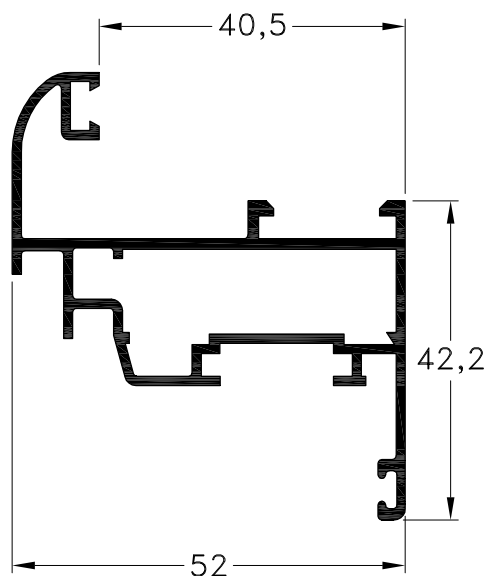
1020661 - Hoja Curva Peso: 0,79 Kg/m. Largo Std.: 6.150 mm.
