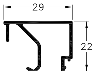
1020646 - Contravidrio Recto 29 mm. Peso: 0,29 Kg/m. Largo Std.: 6.030 mm.
