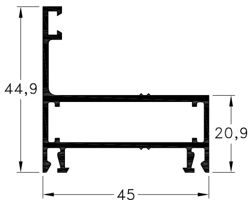
1020676 - Marco Peso: 0,72 Kg/m. Largo Std.: 6.150 mm.
