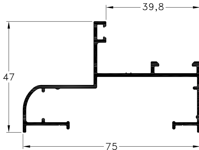
1020910 - Marco de 75 mm. Peso: 0,72 Kg/m. Largo Std.: 6.150 mm.
