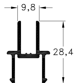
1020642 - Encuentro de Cuatro Hojas Peso: 0,29 Kg/m. Largo Std.: 6.150 mm.
