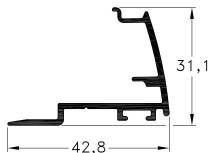
1020363 - Encuentro Central Peso: 0,38 Kg/m. Largo Std.: 6.150 mm.
