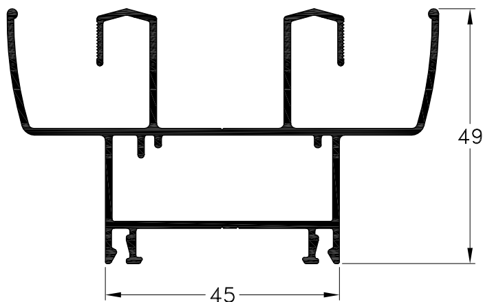
1020360 - Marco a 45° Peso: 1,13 Kg/m. Largo Std.: 6.150 mm.
