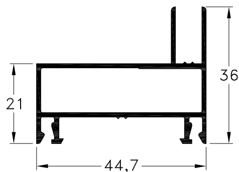
1020655 - Jamba Marco Peso: 0,59 Kg/m. Largo Std.: 6.150 mm.
