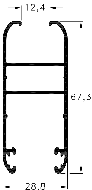
1020361 - Hoja Perimetral V.S. Peso: 0,82 Kg/m. Largo Std.: 6.150 mm.
