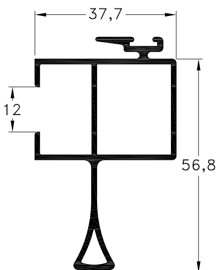
1020677 - Parante Central V.S. con Tirador Peso: 0,79 Kg/m. Largo Std.: 6.150 mm.
