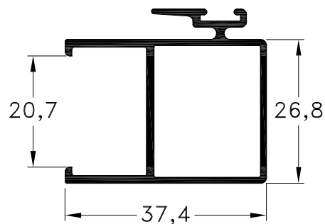
1020664 - Parante Central D.V.H. Peso: 0,51 Kg/m. Largo Std.: 6.150 mm.
