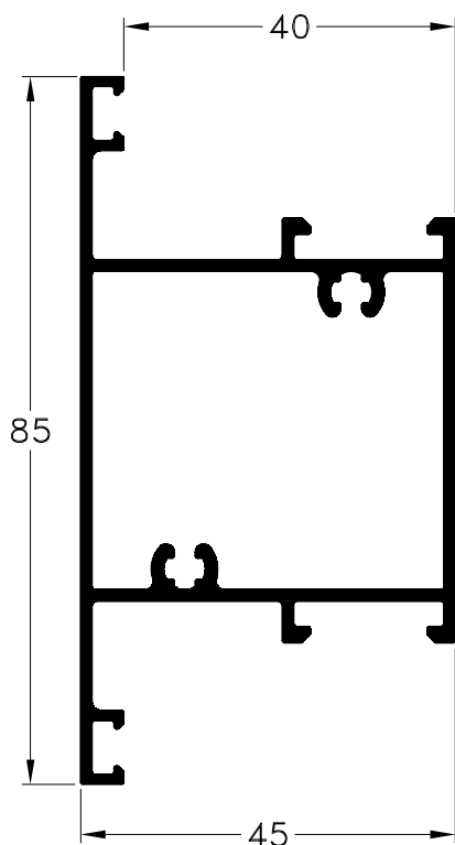
1020615 - Travesaño Peso: 1,09 Kg/m. Largo Std.: 6.030 mm.
