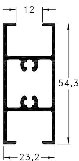
1020638 - Travesaño V.S. Peso: 0,70 Kg/m. Largo Std.: 6.030 mm.
