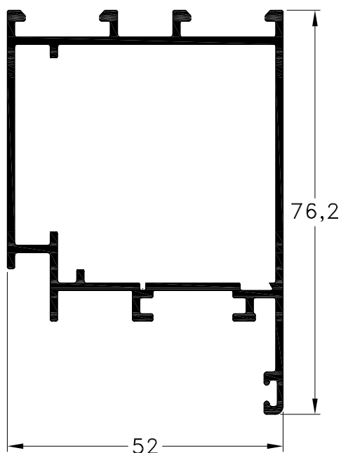
1020356 - Parante Peso: 1,09 Kg/m. Largo Std.: 6.150 mm.
