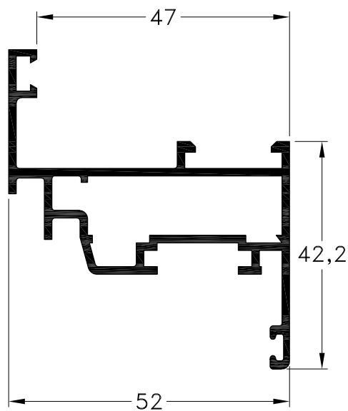
1020635 - Hoja Recta Peso: 0,86 Kg/m. Largo Std.: 6.150 mm.
