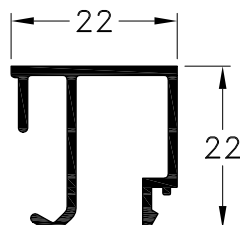
1020633 - Contravidrio Recto 22 mm. Peso: 0,26 Kg/m. Largo Std.: 6.030 mm.
