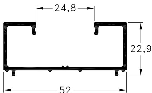
1020936 - Hoja Postigón Celosía Fija Peso: 0,88 Kg/m. Largo Std.: 6.150 mm.
