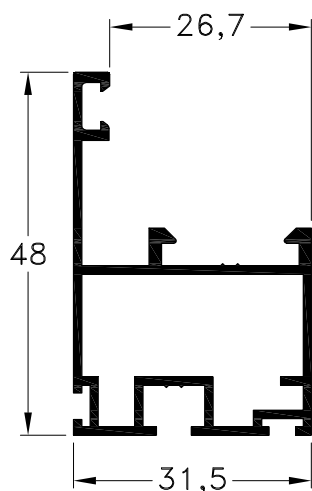
1040507 - Hoja Peso: 0,56 Kg/m. Largo Std.: 6.030 mm.
