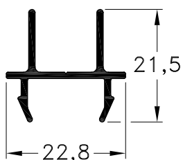
1020365 - Encuentro de Cuatro Hojas Peso: 0,21 Kg/m. Largo Std.: 6.150 mm.
