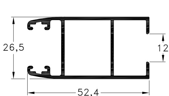
1020653 - Parante Lateral V.S. Peso: 0,64 Kg/m. Largo Std.: 6.150 mm.
