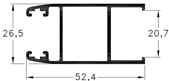
1020665 - Parante Lateral D.V.H. Peso: 0,59 Kg/m. Largo Std.: 6.150 mm.
