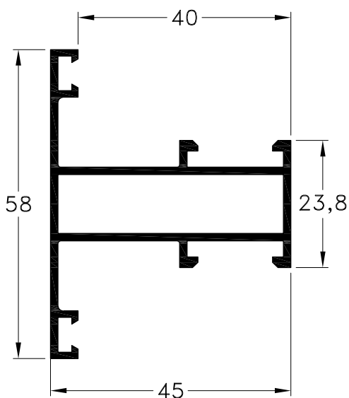
1020629 - Travesaño Angosto para Marco 1020668 Peso: 0,77 Kg/m. Largo Std.: 6.030 mm.
